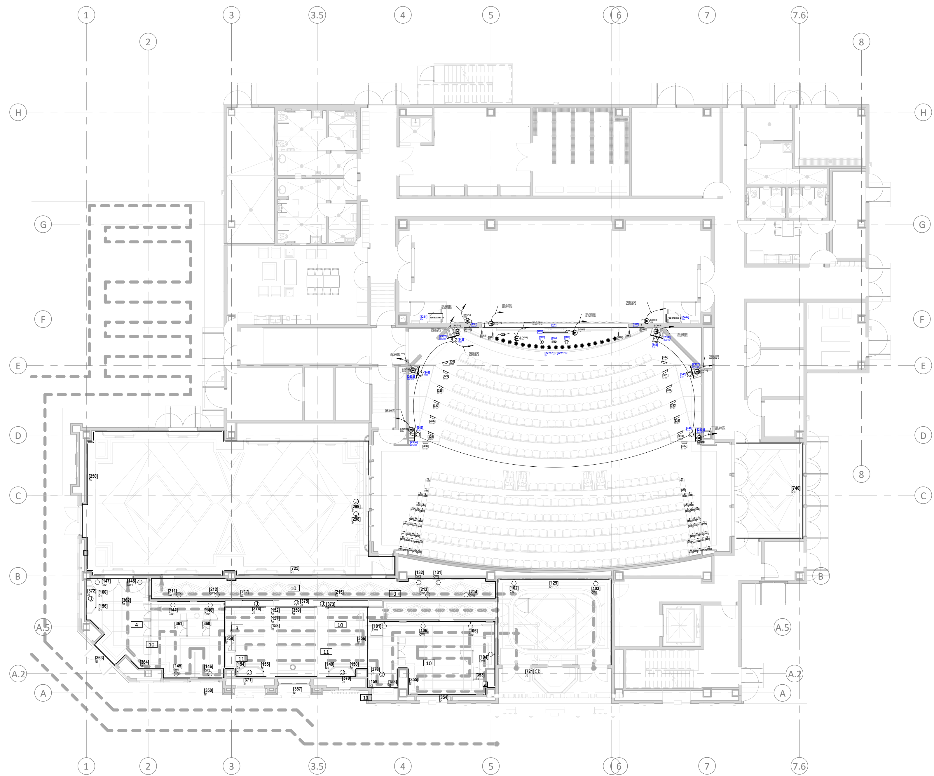
首层平面图 - 主题灯光 1 FLOOR PLAN - THEMED LIGHTING TL122f
