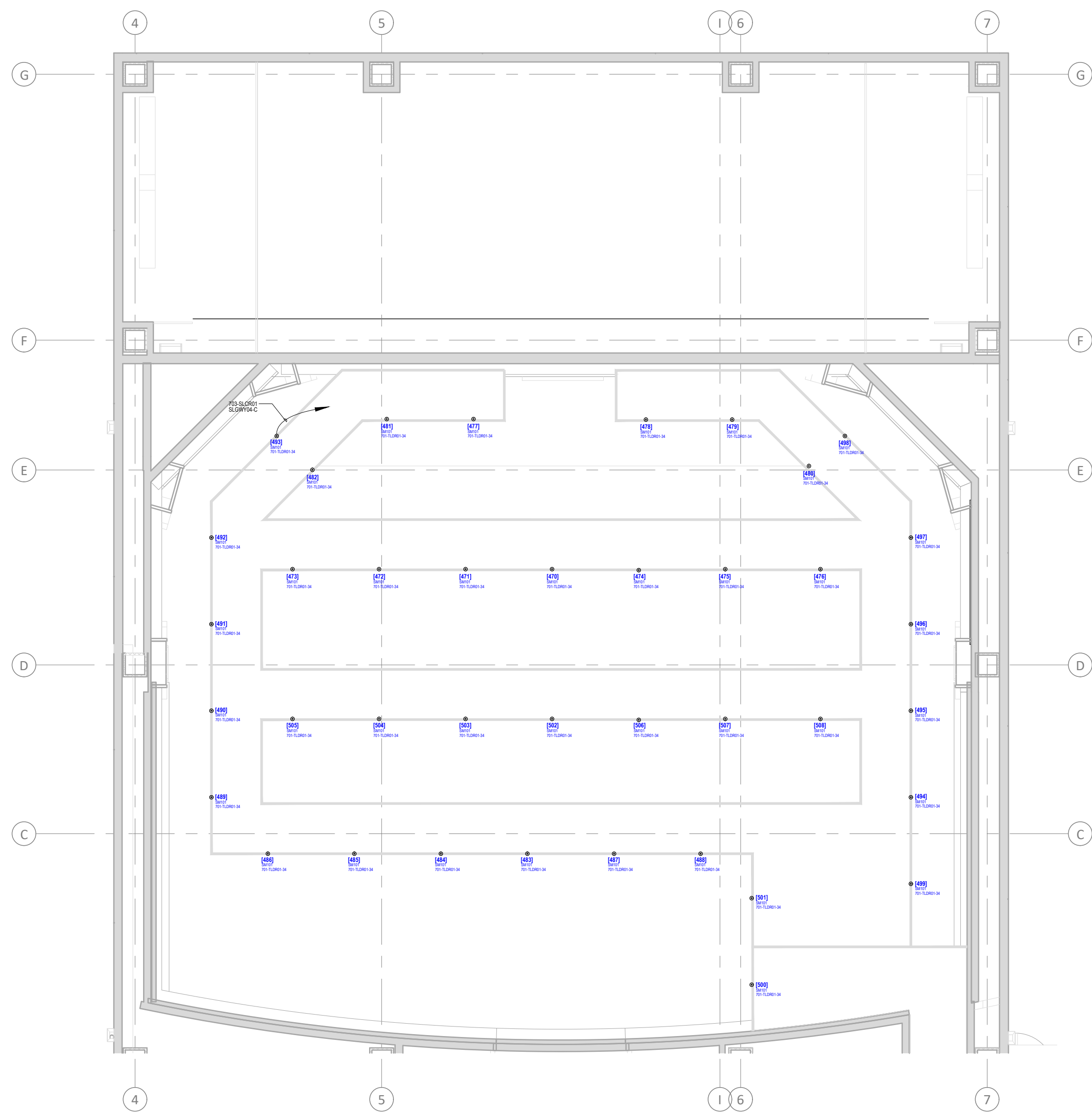
马道平面图 - 主题灯光 CATWALK PLAN - THEMED LIGHTING 1 TL131f
